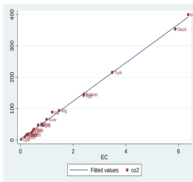
نمودار ۳- پراکنش متوسط انتشار آلودگی ( \text{CO}_2 ) در مقابل متوسط مصرف انرژی (EC) منبع: (World Bank, 2015)
