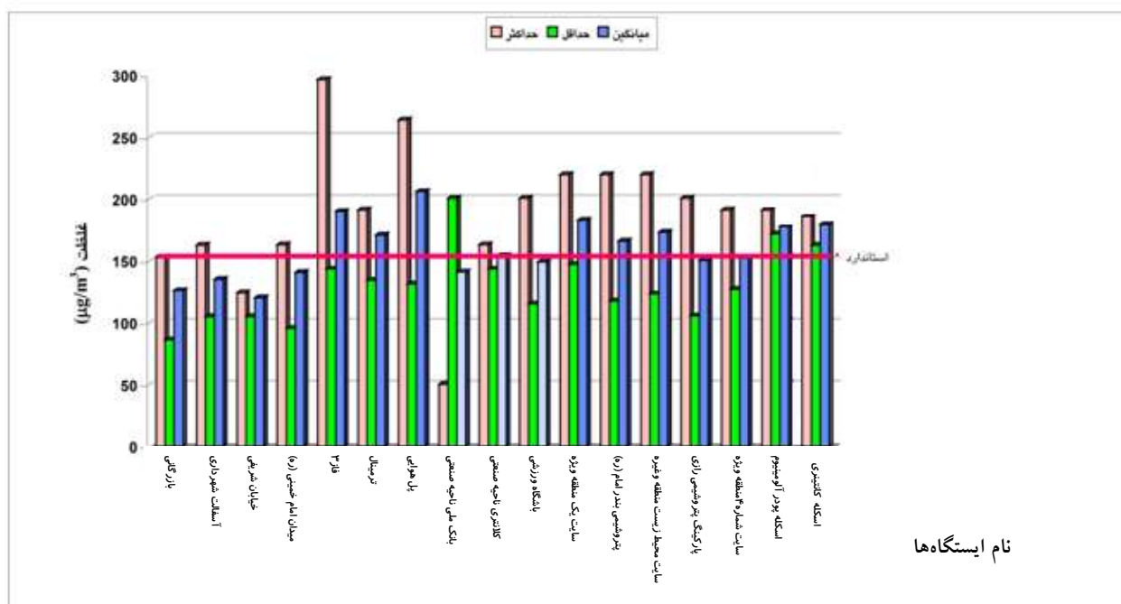
نمودار ۸- حداکثر، حداقل و میانگین پارامتر آلاینده ذرات معلق اندازه‌گیری شده در مراحل نمونه‌برداری هوای محیطی منبع: (یافته‌های نگارندگان)
